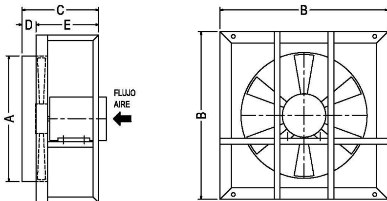
MODELO AXM - ARREGLO 4 - TRANSMISION DIRECTA
