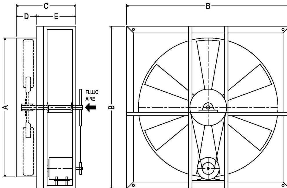
MODELO AXM - ARREGLO 9 - TRANSMISION POLEAS Y BANDAS
